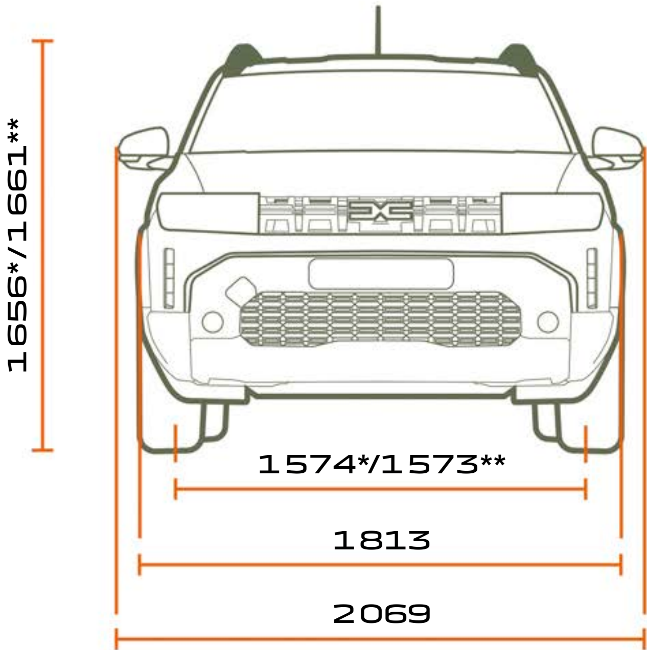
VUE AVANT
